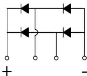
线路图 Circuit
