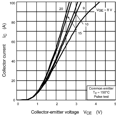
Fig. 8.3 I_C - V_{CE}
