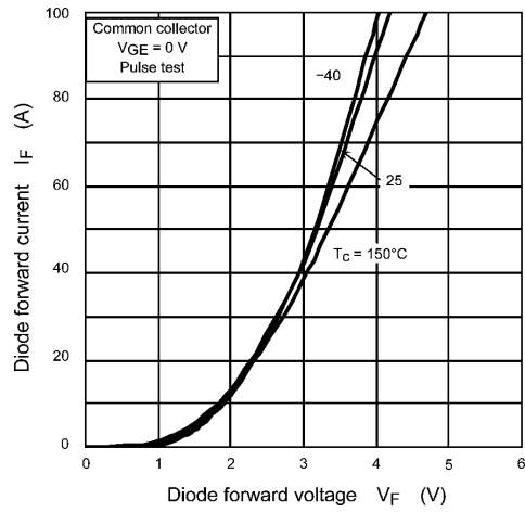
Fig. 8.10 I F - V F
