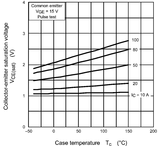
Fig. 8.4 V_{CE(sat)} - T_C
