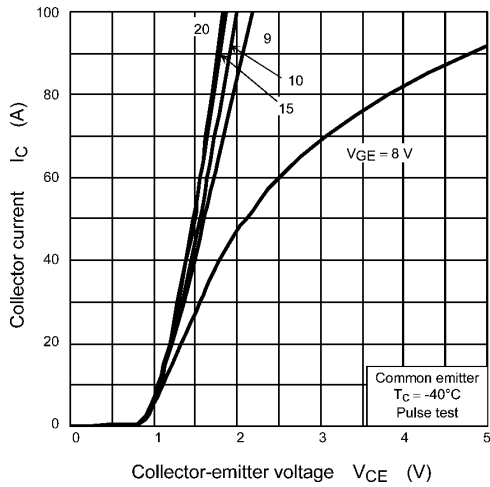
Fig. 8.1 I_C - V_{CE}
