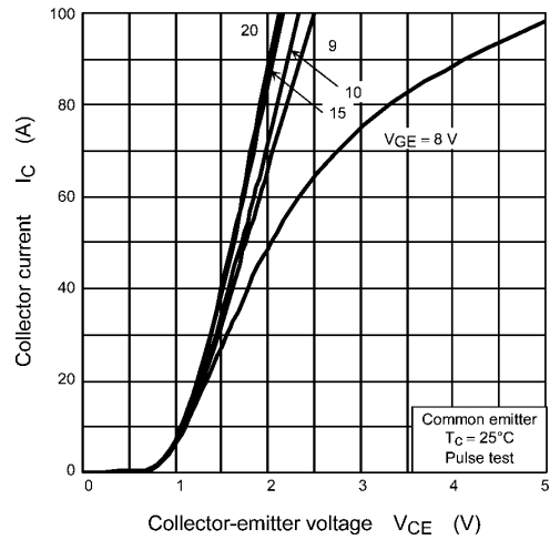
Fig. 8.2 I_C - V_{CE}
