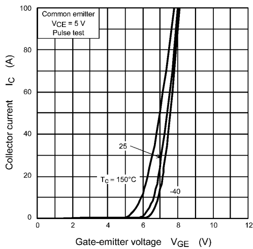
Fig. 8.5 I_C - V_{GE}
